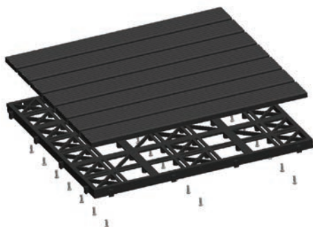
Conjunto Deck Modular Plástico
